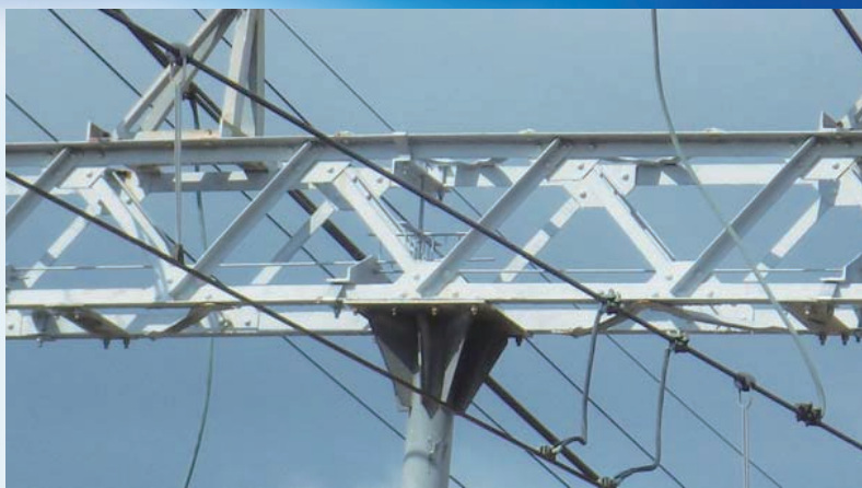
鳥害防止金具トラス上面用及び下面用施工後写真
