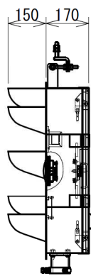
側面図
